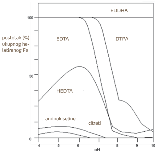
Utjecaj pH na različite oblike helata
